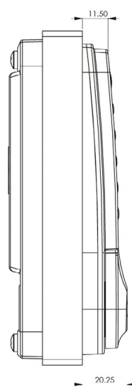
RFID NIMBUS SEMI-FLUSH FIT
